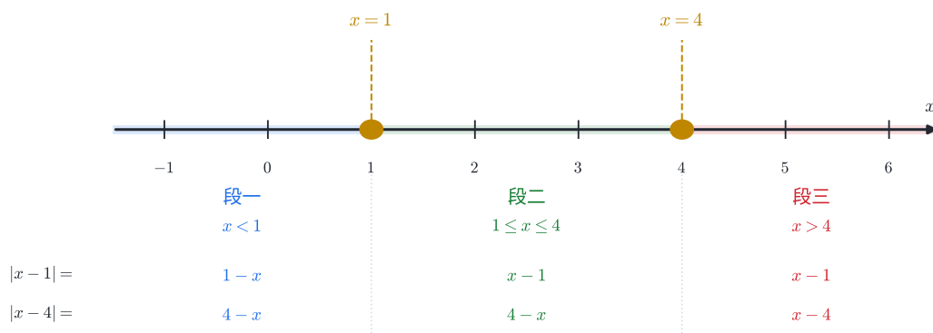
圖 1-4：分段討論法示意（以 |x-1| + |x-4| 為例）。兩個變號點 x=1 、 x=4 把數線切成三段；下方表格列出每一段內 |x-1| 與 |x-4| 各自如何去掉絕對值符號。例如段一（ x < 1 ）兩個內部皆為負，故 |x-1| = 1-x 、 |x-4| = 4-x ；段二（ 1 \leq x \leq 4 ）則 |x-1| = x-1 、 |x-4| = 4-x 。
